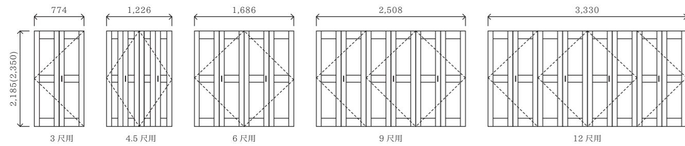
規格サイズ (収納扉)
